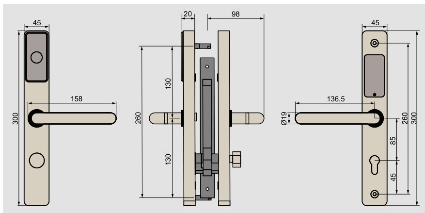
Cerradura mecánica de emergencia oculta tras tapa en la parte frontal.
