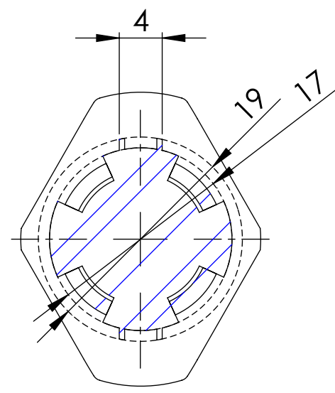
CORTE A-A
